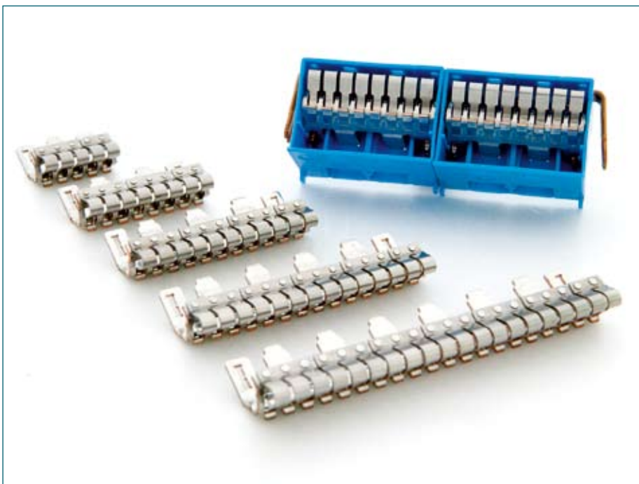
Schraubenlose Klemmleisten in unterschiedlichen Varianten fertigt Bogner auf einem Multicenter ohne Werkzeugwechsel.
